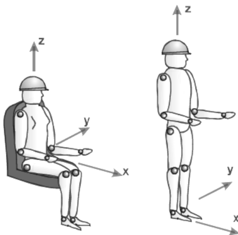
Figur 19: Måleretninger for helkroppsvibrasjoner (3).
