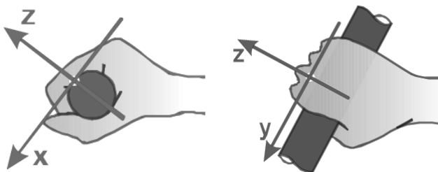
Figur 8: Måleretninger for hånd- og armvibrasjoner (2).
