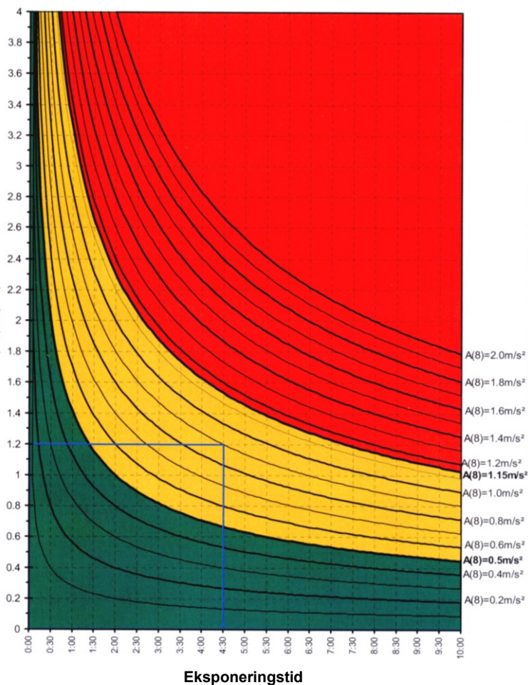
Figur 22: Eksponeringsgraf for helkroppsvibrasjoner.
