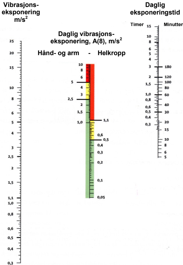
Figur 23: Nomogram for beregning av daglig vibrasjonseksposering (1).
